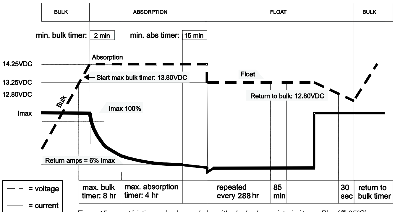
Figure 15: caractéristiques de charge de la méthode de charge à trois étapes Plus (@ 25°C)
